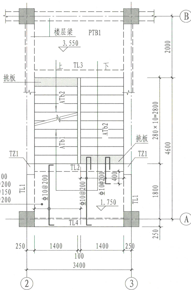
▽1.750~▽3.550楼梯平面图
