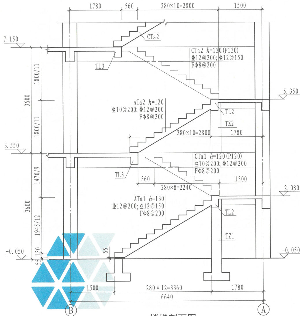
楼梯剖面图
