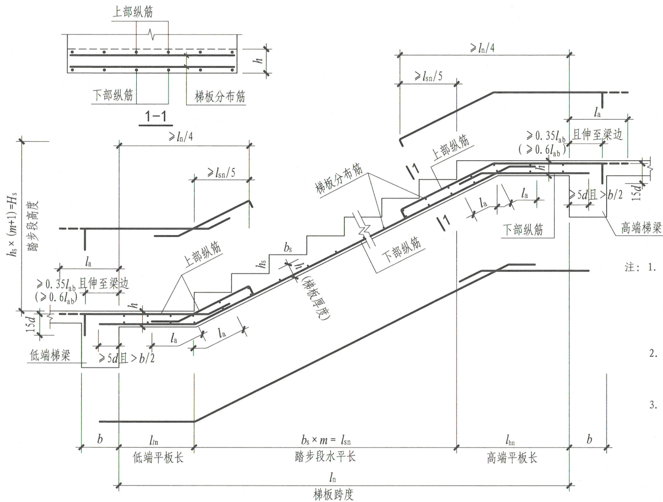
DT型楼梯板配筋构造
