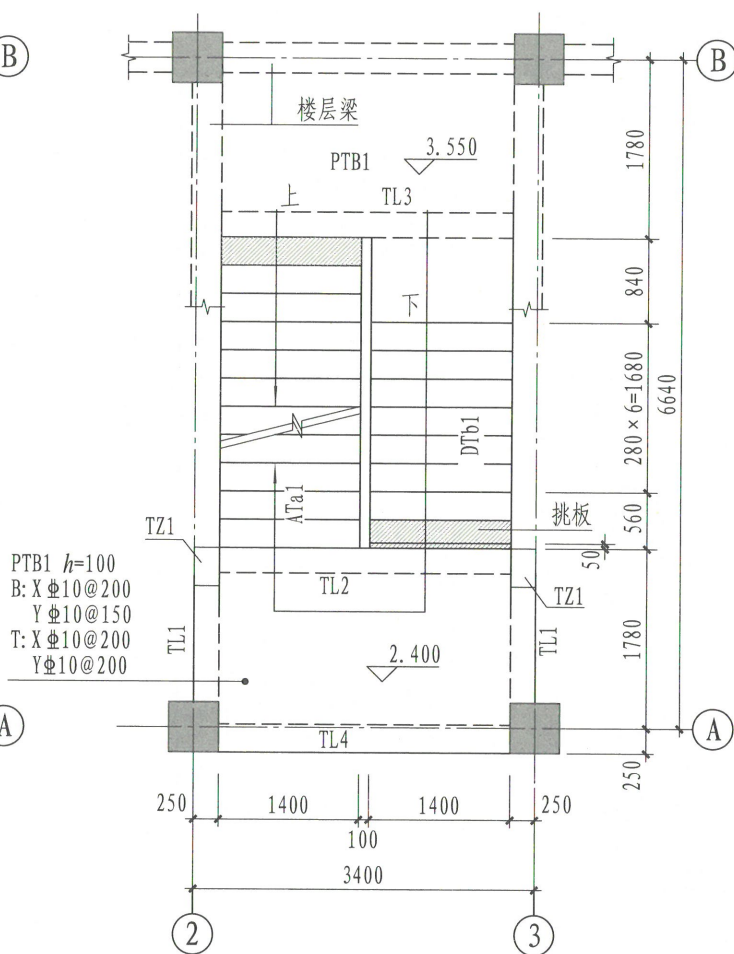
▽2.400~▽3.550楼梯平面图
