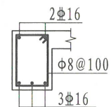
TL2、TL3、TL4 250 × 400
