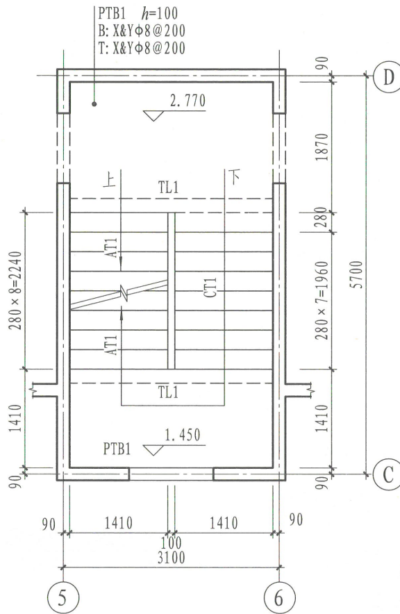
▽1.450~▽2.770楼梯平面图
