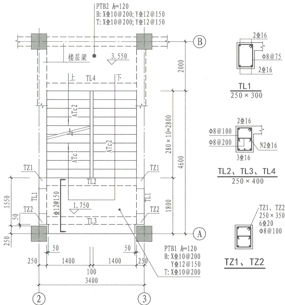
▽1.750~▽3.550楼梯平面图
