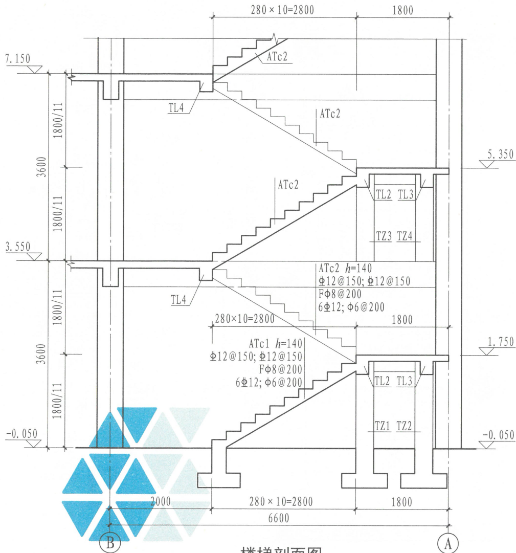
楼梯剖面图 (局部示意)
