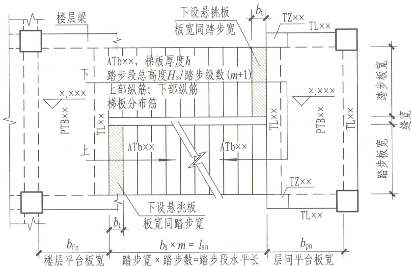
图2 ▽x.xxxx~▽x.xxxx楼梯平面图 (ATb型注写方式)
