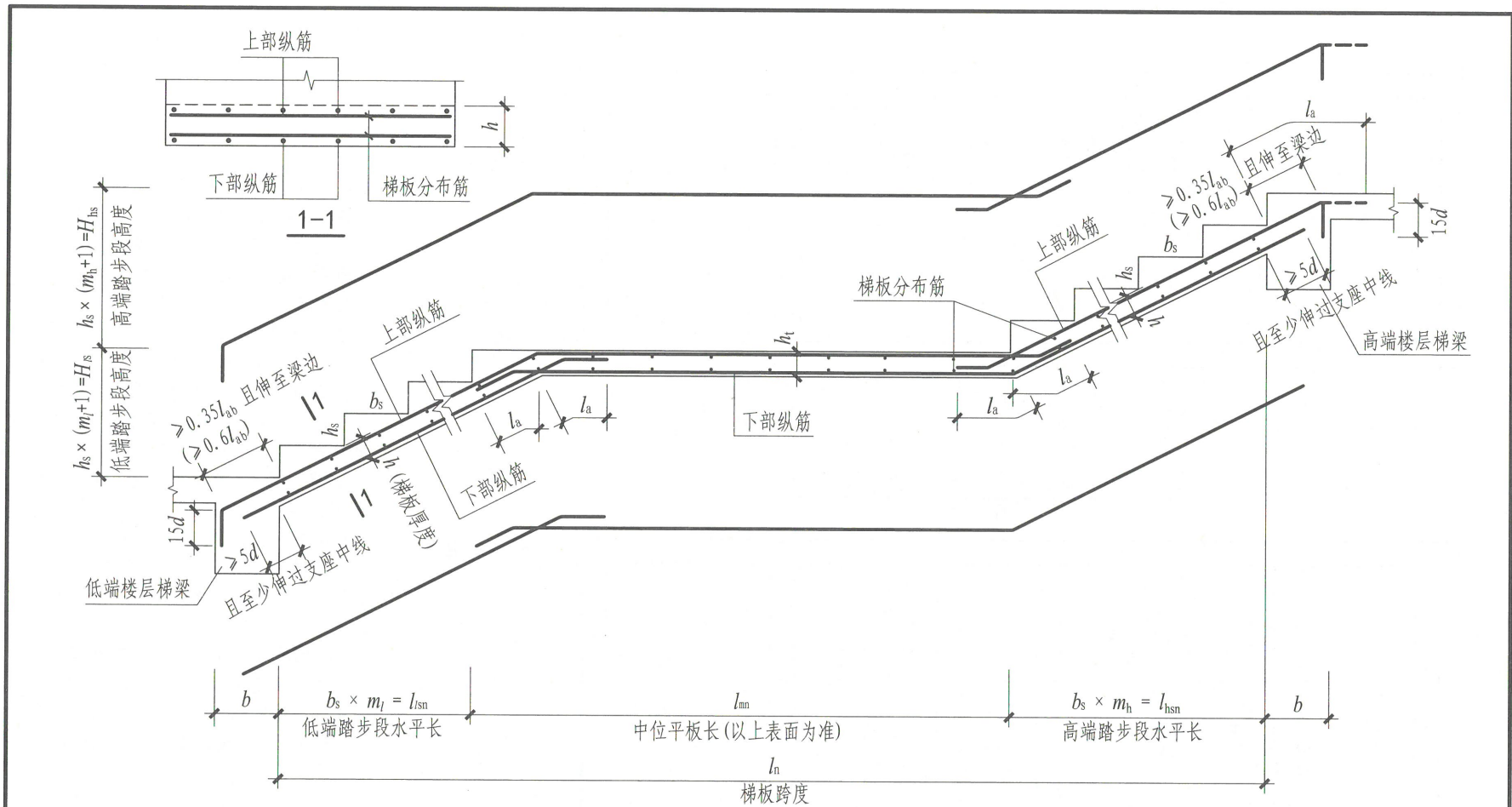
ET型楼梯板配筋构造
