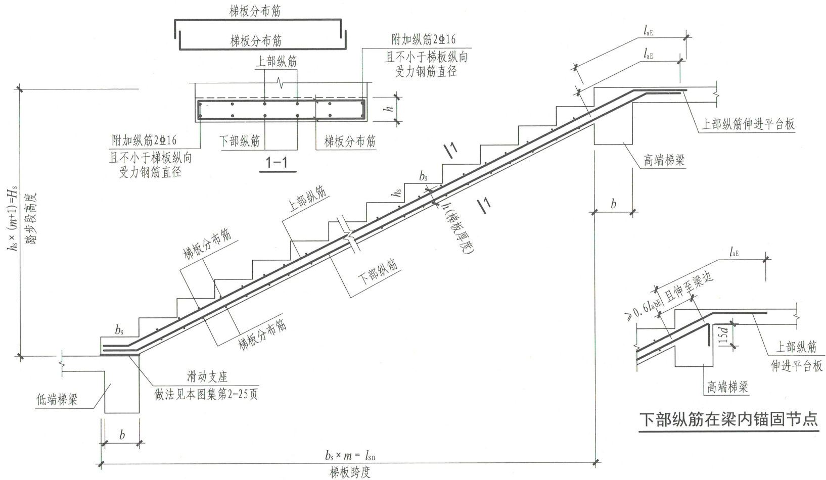
ATa型楼梯板配筋构造
