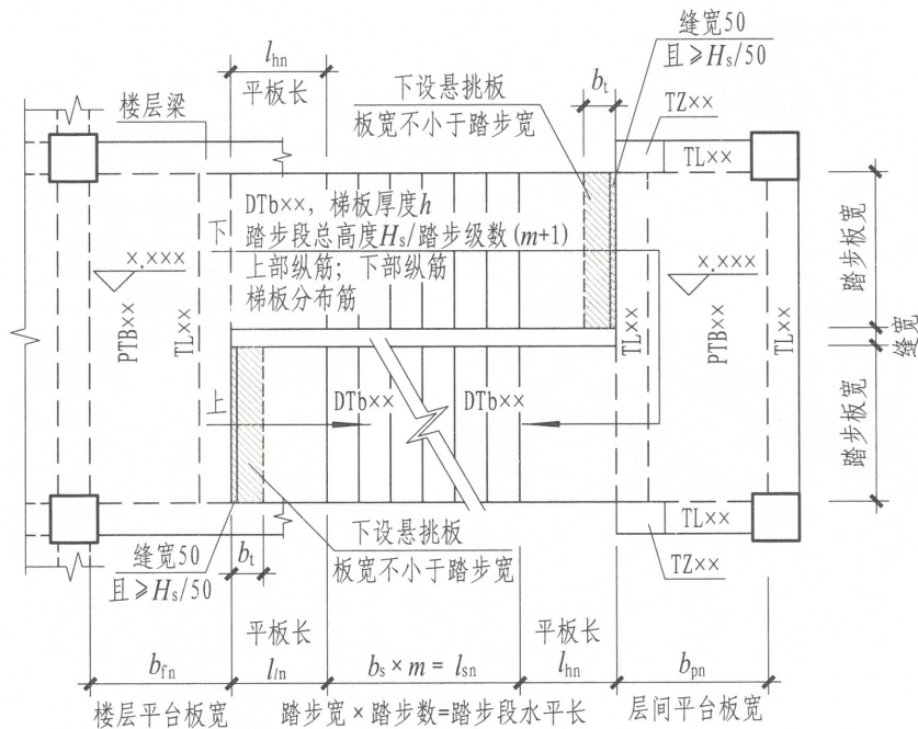
图1 \nabla x. xxx \sim \nabla x. xxx 楼梯平面图 (DTb型注写方式)
