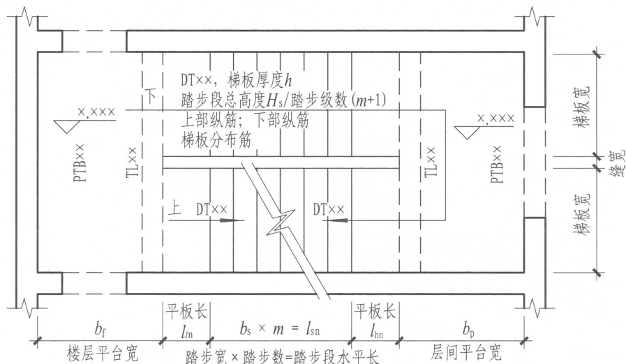
图1 ∇x.xxx~∇x.xxx楼梯平面图 (注写方式)
