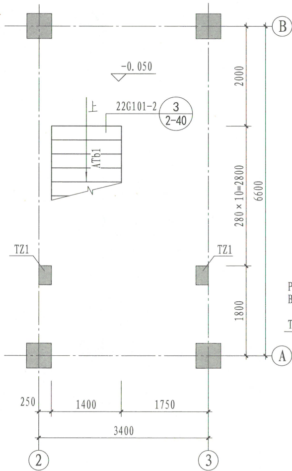
▽-0.050楼梯平面图
