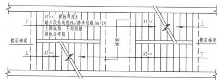
图4 剪刀楼梯
