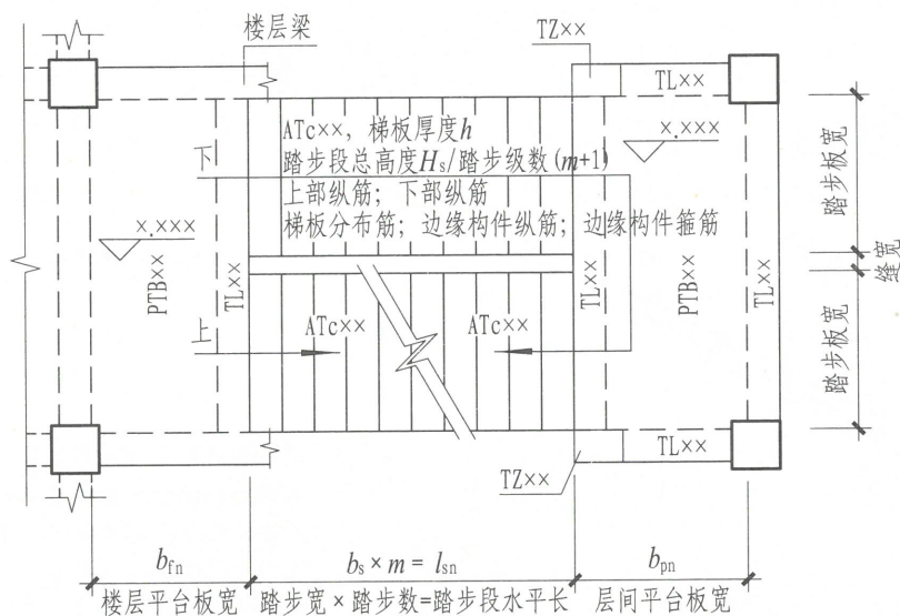
图1 ▽x.xxx~▽x.xxx楼梯平面图
