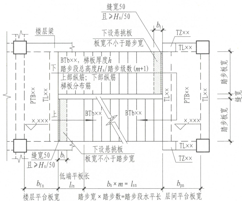
图1 \nabla x.xxx \sim \nabla x.xxx 楼梯平面图
