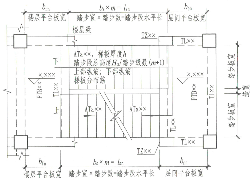
图1 ▽x.xxxx~▽x.xxxx楼梯平面图 (ATa型注写方式)
