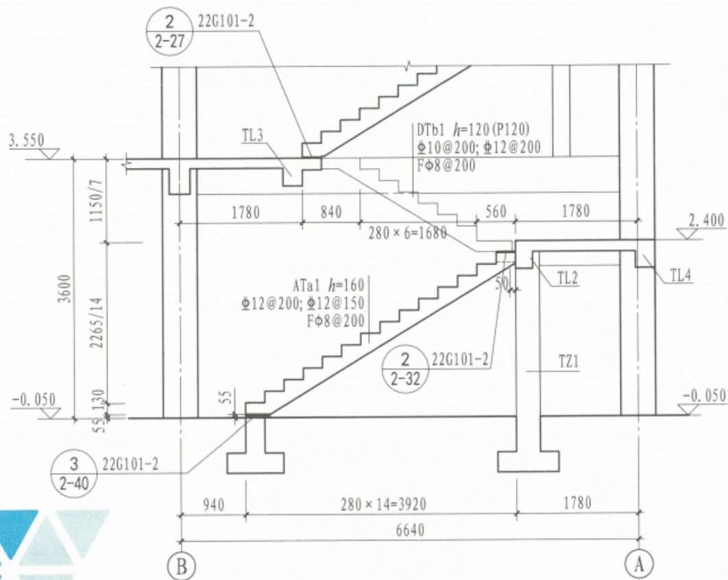
楼梯剖面图
