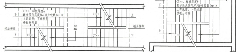
图4 剪刀楼梯
