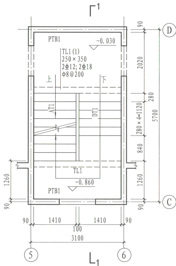
▽-0.860~▽-0.030楼梯平面图
