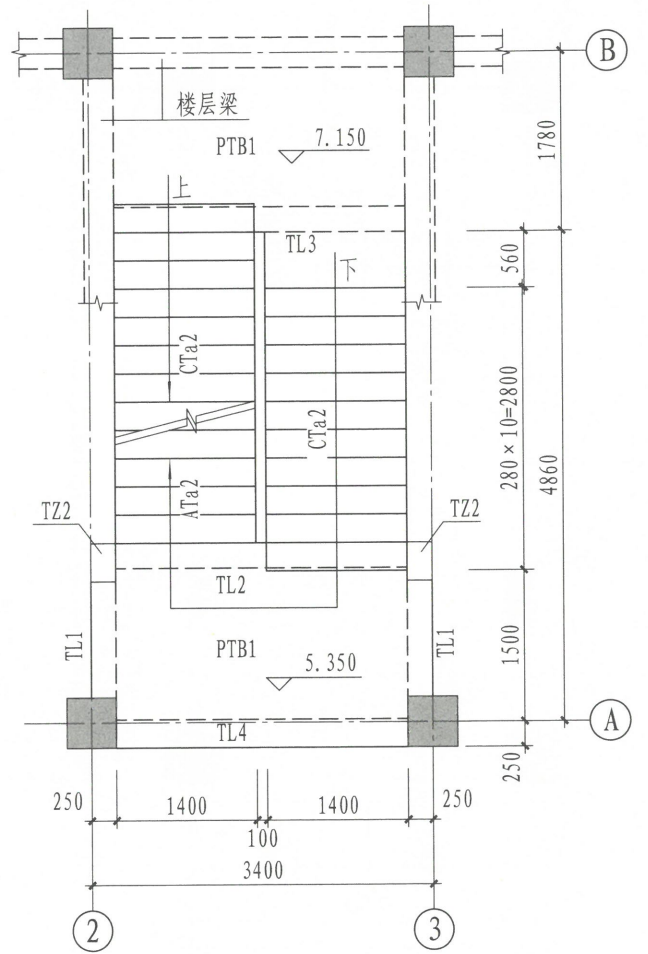
▽5.350~▽7.150楼梯平面图
