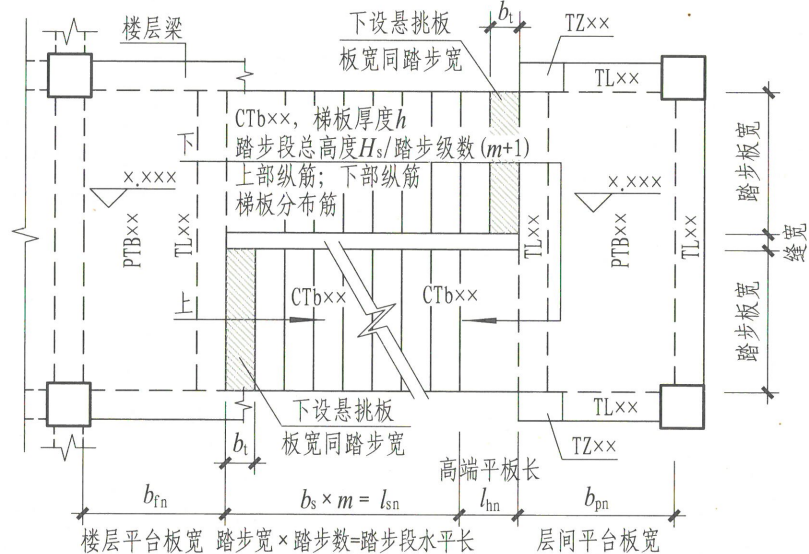
图2 \nabla x. xxx \sim \nabla x. xxx 楼梯平面图
