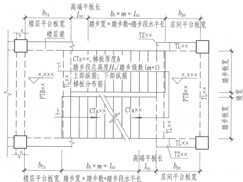
图1 \nabla x. xxx \sim \nabla x. xxx 楼梯平面图
