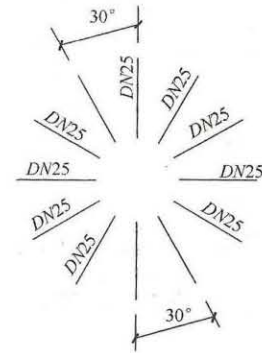
图 4.5.13 管径（压力）的标注位置示例
