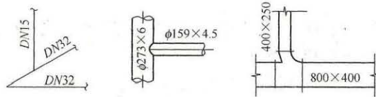
图 4.5.12 管道截面尺寸的画法
