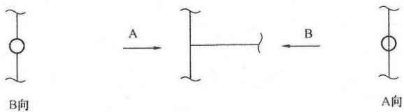
图 4.6.3 单线管道分支的画法
